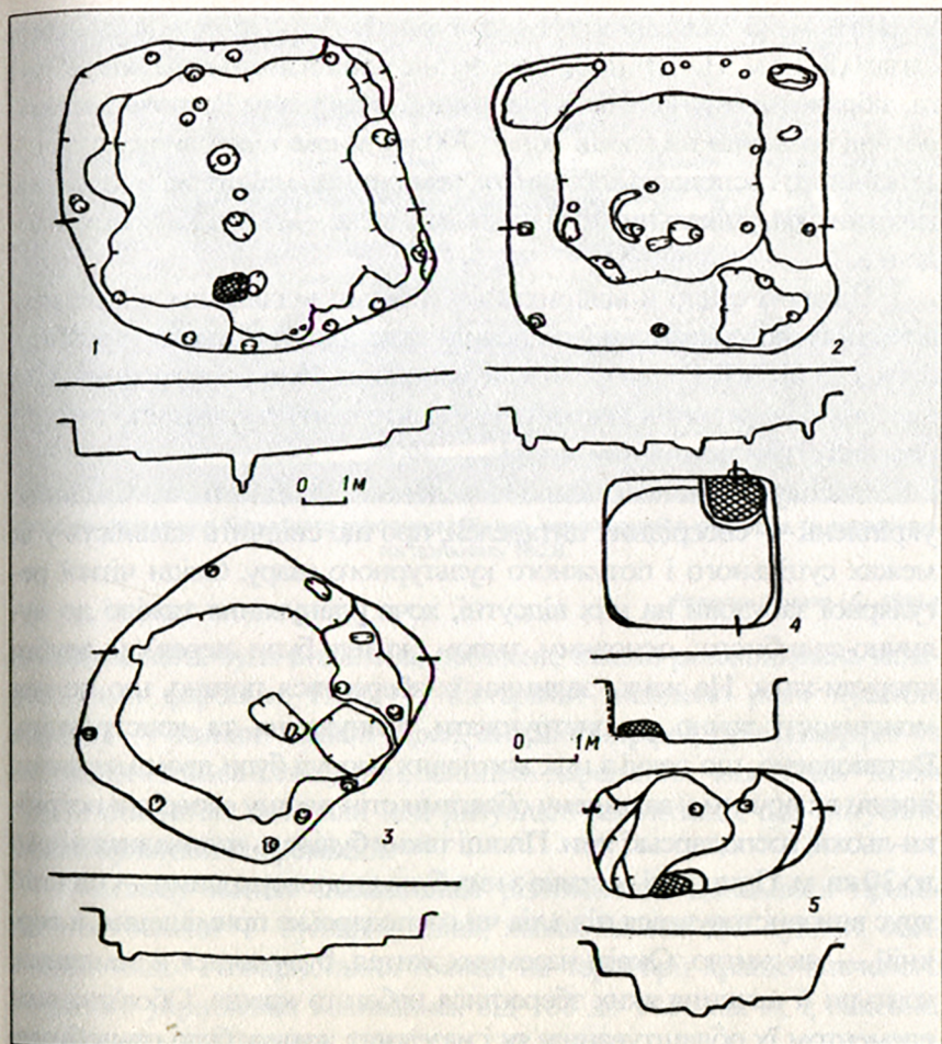
Плани та перетини землянок Західного (1-3) і Східного (4-5) укріплень.
