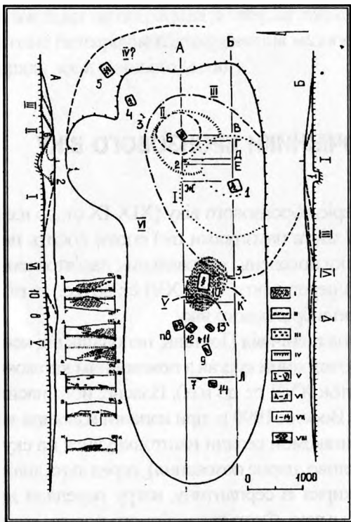
Рис.28. Михайлики, с. "Довгий" курган культури багатоваликової кераміки та зрубної культури. Розкопки Л.Лугової і Ю.Шилова, 1985 р. План.
