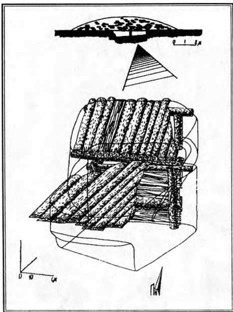
Рис.41. Карпусі . Курган № 2. Схематичний перетин насипу та реконструкція поховальної споруди передскіфського часу.
